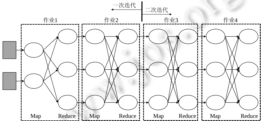
Fig.10 MapReduce for PageRank with two iterations 图 10 MapReduce 处理 PageRank 问题两次迭代
