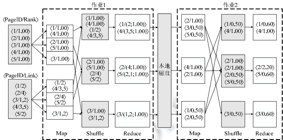
Fig.9 MapReduce for PageRank with one iteration 图 9 MapReduce 处理 PageRank 问题一次迭代
